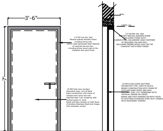
DOOR SECTION DETAILS A
