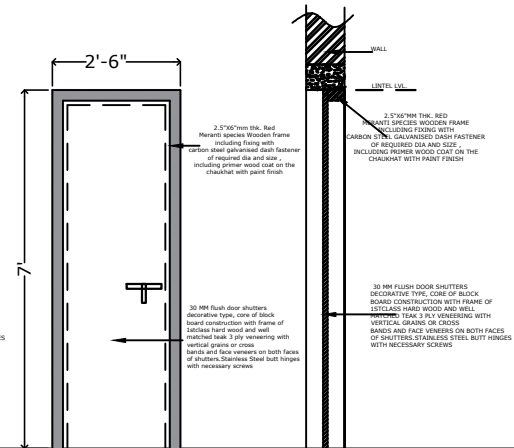
DOOR SECTION DETAILS C
