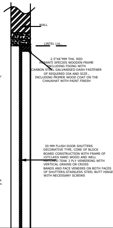
DOOR SECTION DETAILS B
