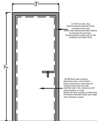
D1 (3'-0"x7'-0") (B)
